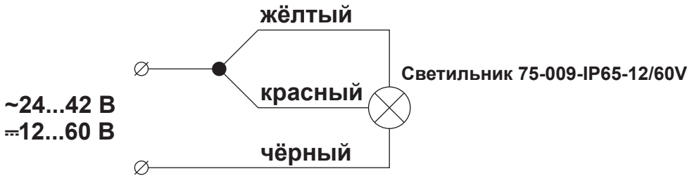
Рисунок 2. Схема подключения светильника 75-009-IP65-12/60V к питающей сети
